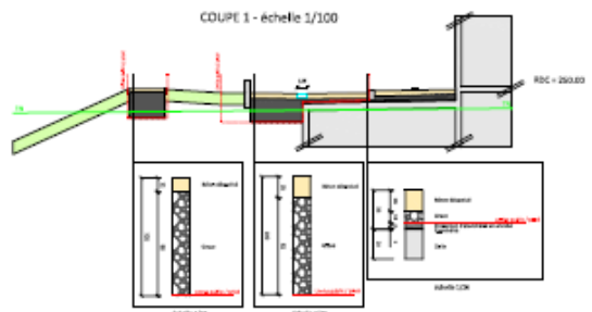
COUPE 1 - échelle 1/100
